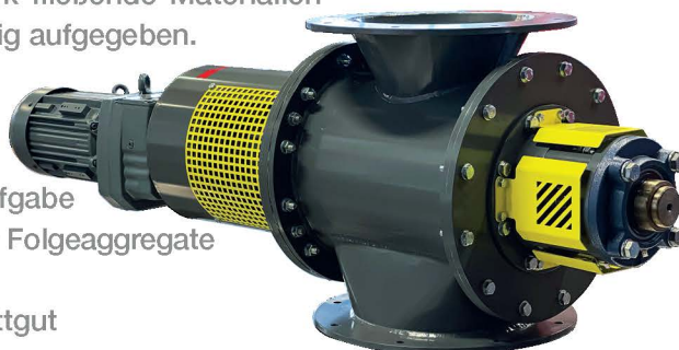
Zellenradschleuse
