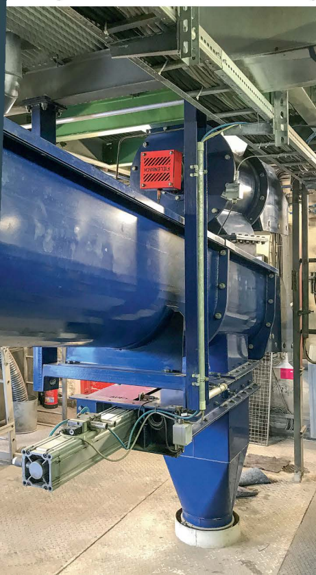
Trogscneckenförderer zur Ascheverladung
